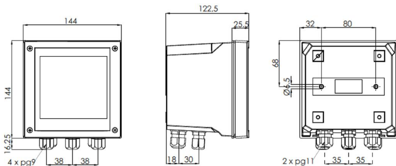
VERSIÓN DE MONTAJE EN PARED (144 x 144 x 122,5 mm.)
