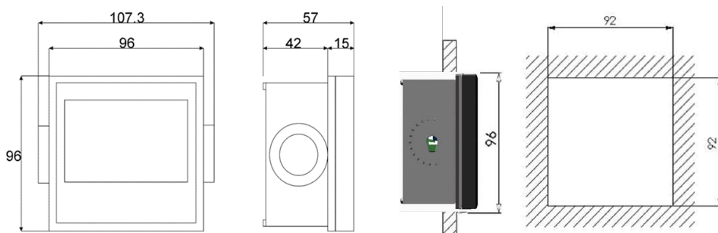
VERSIÓN DE MONTAJE EN PANEL (96 x 96 x 42 mm.)
